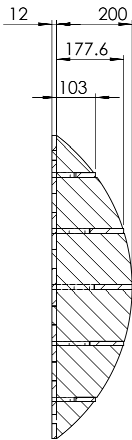
SCHNITT A-A
